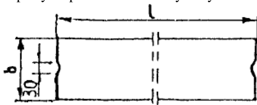
Rys. 1. Wymiarowanie krawężników
